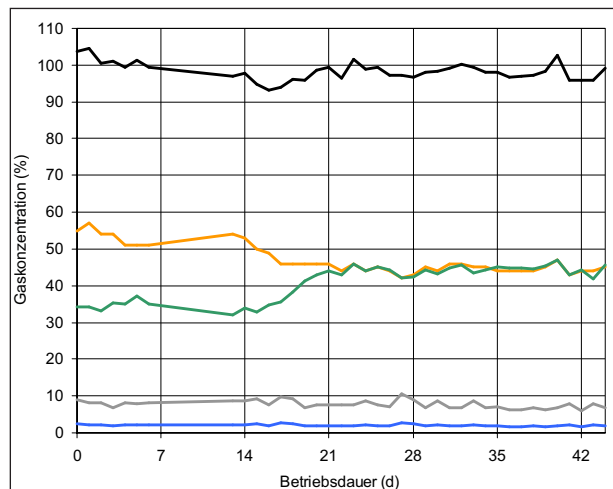
Grafik: Gaszusammensetzung
